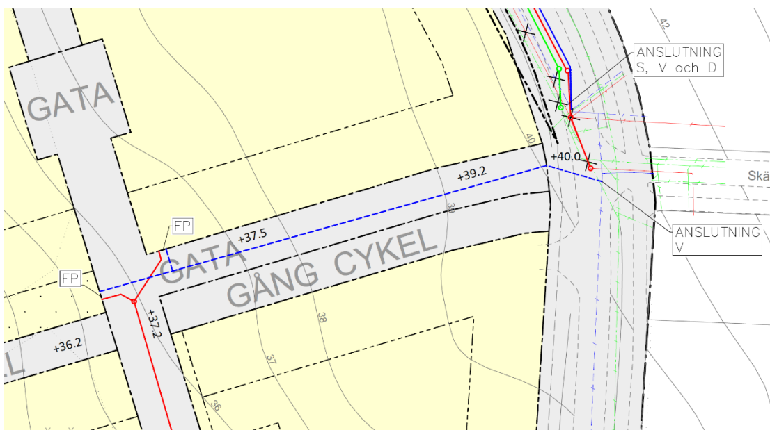
Figur 3 Föreslagen ledningssträckning enligt Bilaga 2.
