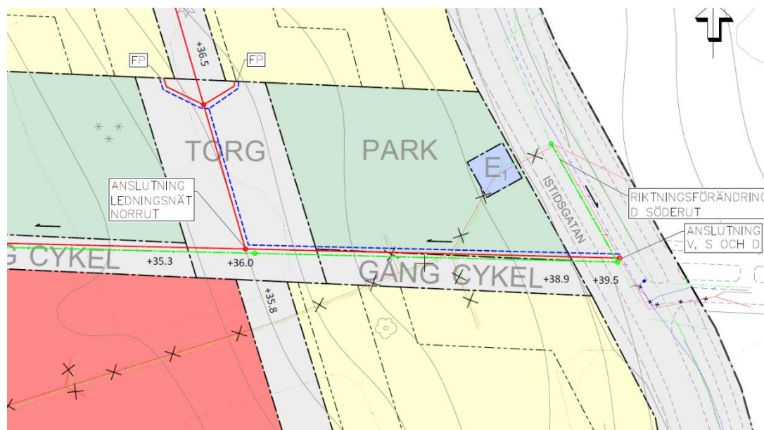
Figur 4 Föreslagen ledningssträckning Mitten gatans östra del enligt Bilaga 3
